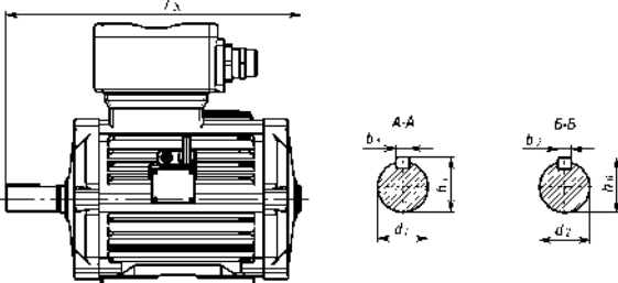
Рисунок Е.1 – Габаритные и установочные размеры
