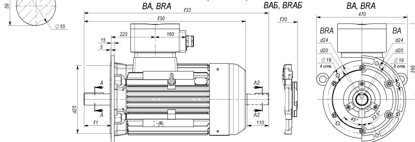
* Габаритный чертеж IM30x1; IM30x2
