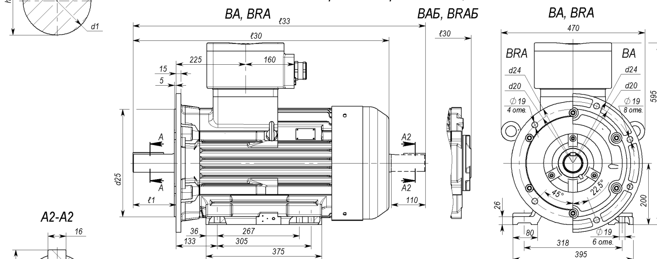
* Габаритный чертеж IM30x1; IM30x2
