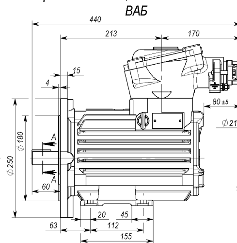
Габаритный чертеж BA100S2, S4 IM30x1
