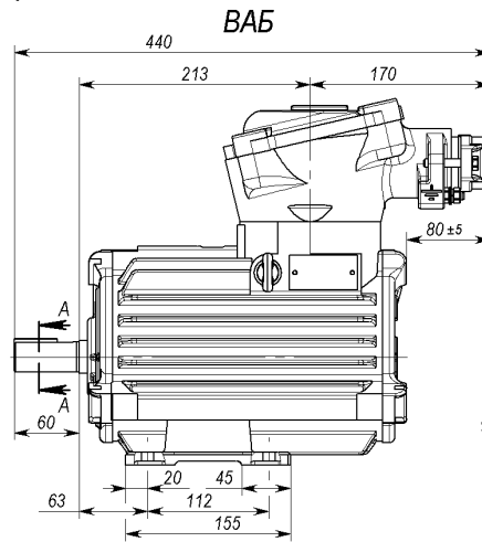
Габаритный чертеж BA100S2, S4 IM20x1
