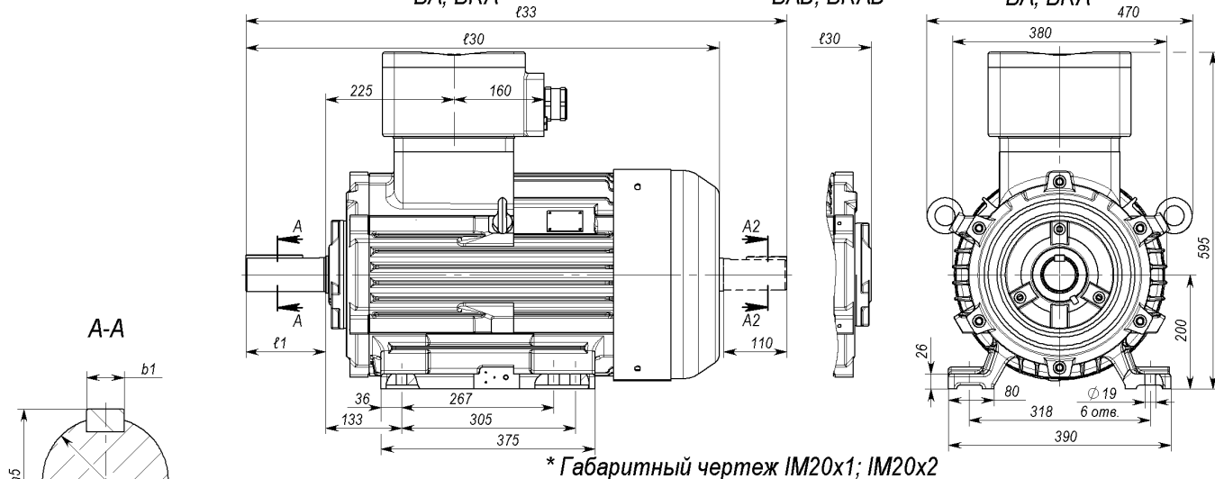
* Габаритный чертеж IM10x1; IM10x2 BA, BRA BAБ, BRAБ
