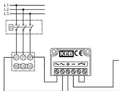
Схема подключения от контактов в коробке выводов двигателя. ( Не допустима при работе от преобразователя частоты)
