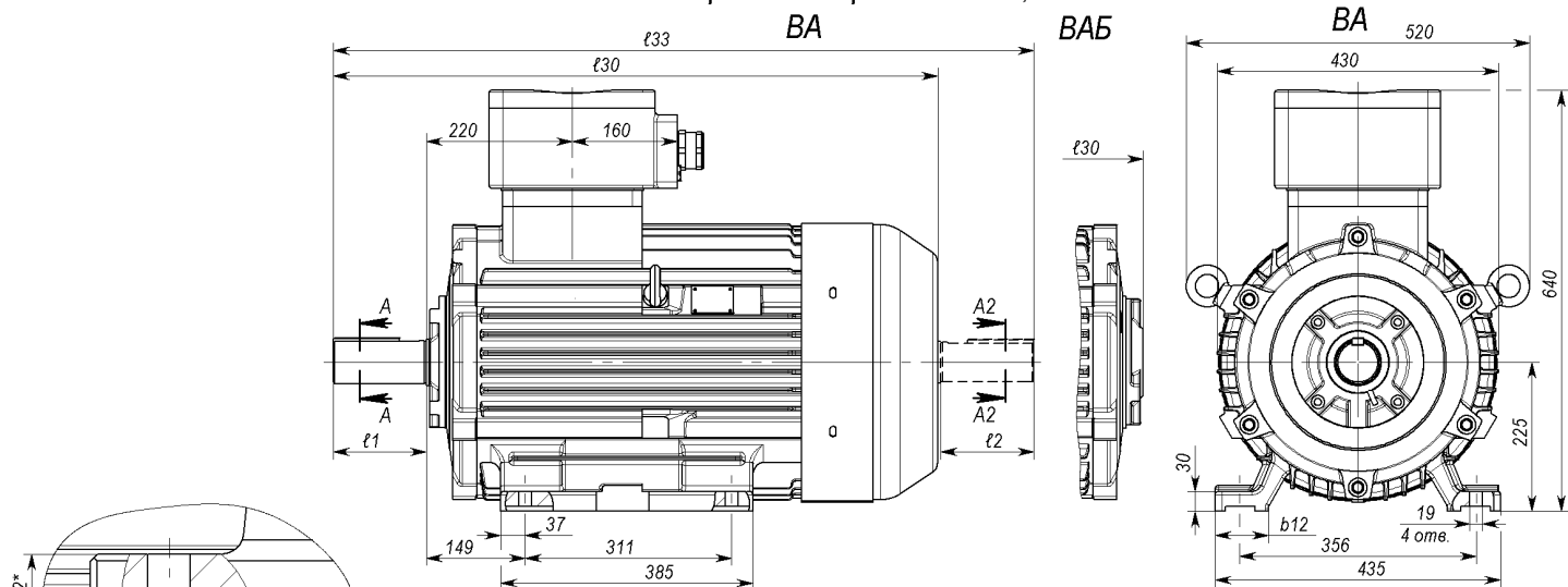
Габаритный чертеж IM20x1; IM20x2
