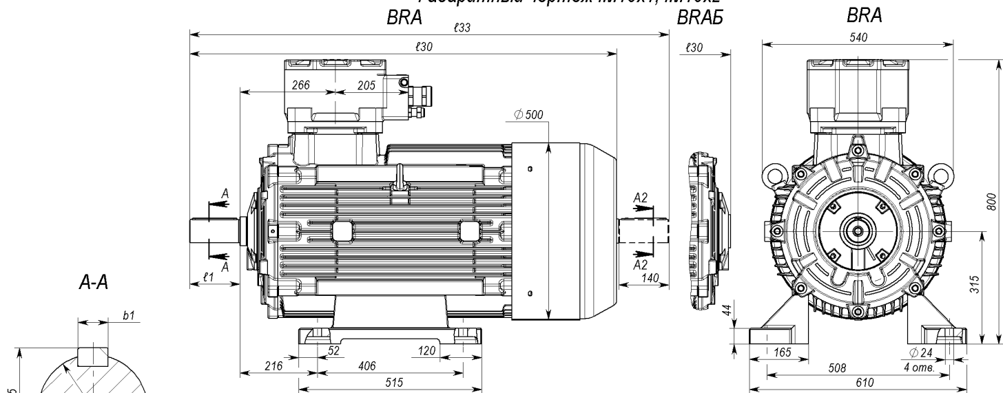
Габаритный чертеж IM20x1; IM20x2
