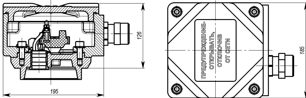
Коробка выводов двигателей ВА (BRA) 132; 160; 180. (Вид взрывозащиты 1Exde ПВ/ПС)
