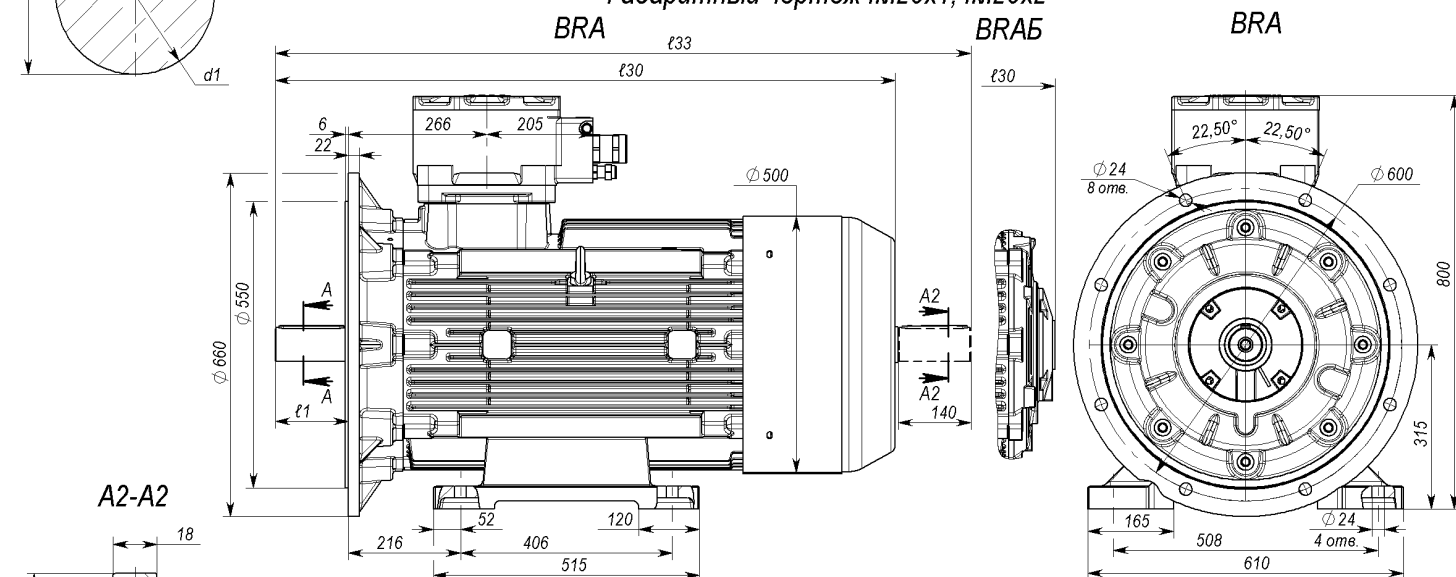
Габаритный чертеж IM30x1; IM30x2
