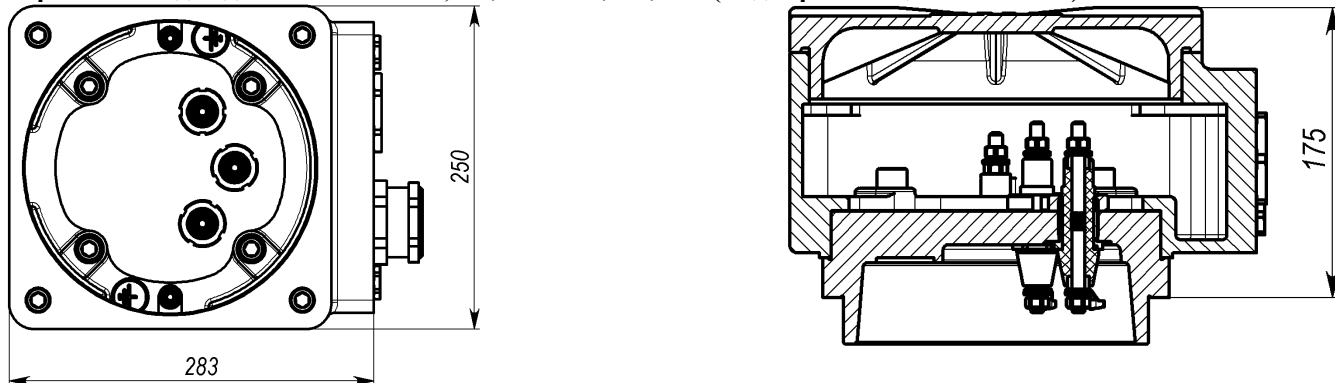
Коробка выводов двигателей ВА200,225; BRA200,225;250. (Вид взрывозащиты 1Exd ПС)
