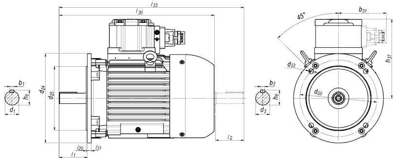
Возможные варианты исполнений взрывозащищенных двигателей
