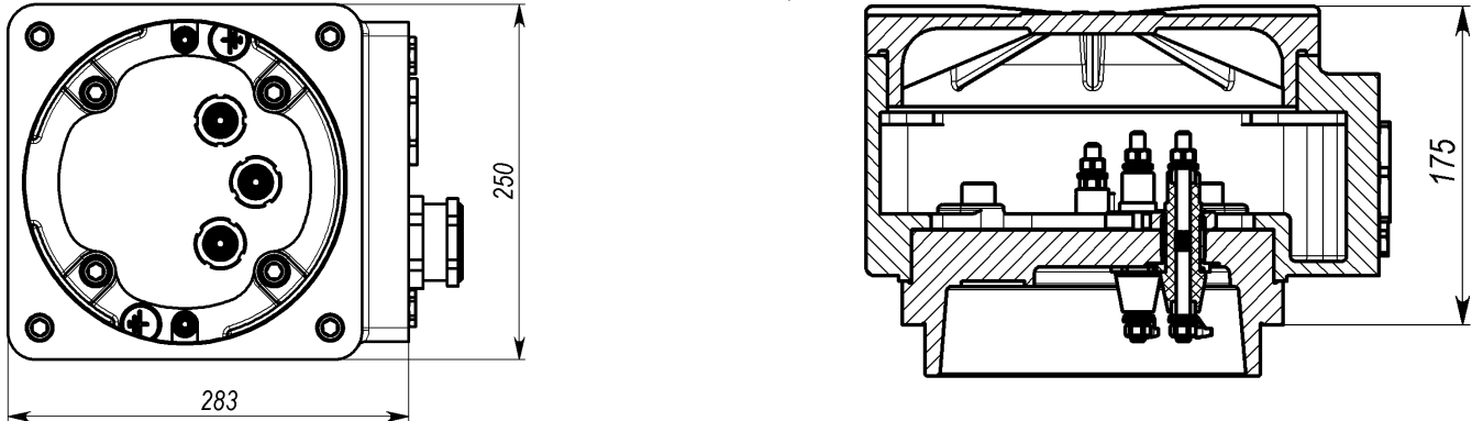
Коробка выводов двигателей ВА200,225; BRA200,225;250. (Вид взрывозащиты 1Exd IIС)
