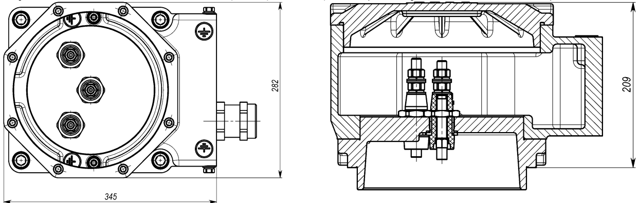
Коробка выводов двигателей ВА 250, 280S; BRA280, 315S. (Вид взрывозащиты 1Exd IIС)
