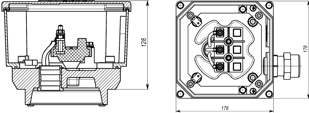
Коробка выводов двигателей ВА (BRA) 132; 160; 180. (Вид взрывозащиты 1Exde IIВ/IIС)
