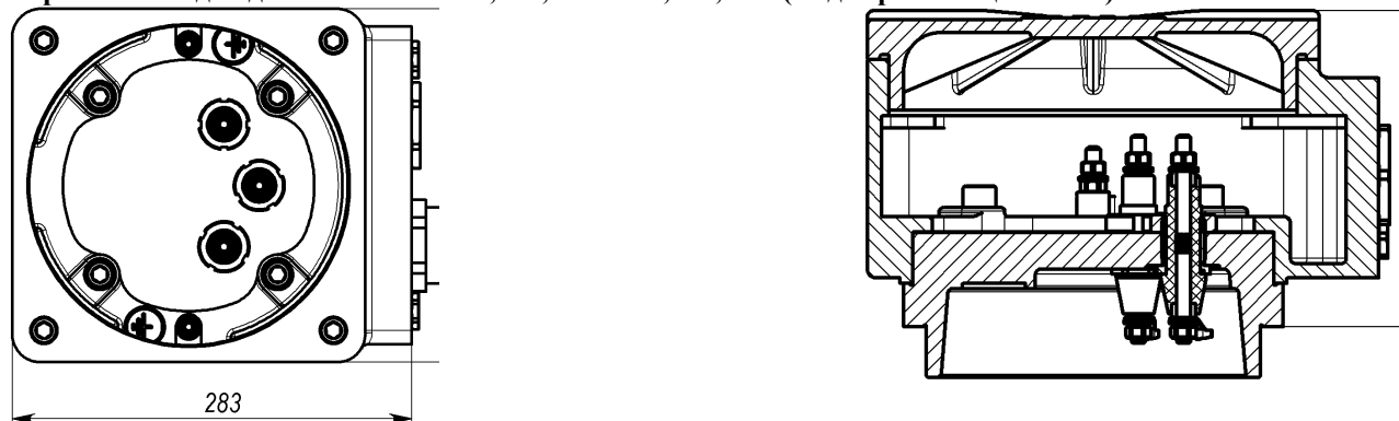
Коробка выводов двигателей BA200,225; BRA200,225;250. (Вид взрывозащиты «d»)
