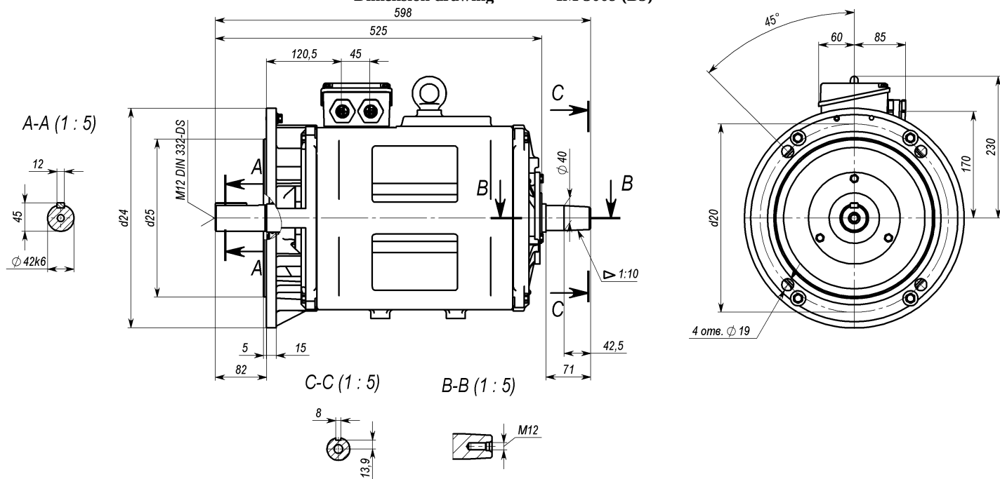
Габаритный чертеж Dimension drawing
