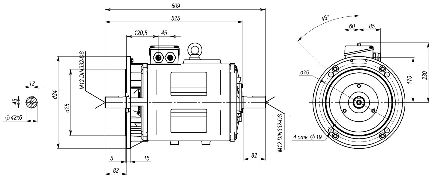
Габаритный чертеж Dimension drawing
