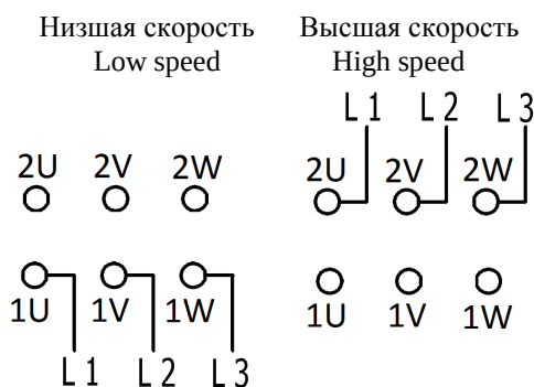
Рис.2 - Схема подключения 2-скоростного двигателя с двумя отдельными обмотками или одной обмоткой по схеме «YYY/YYY»
