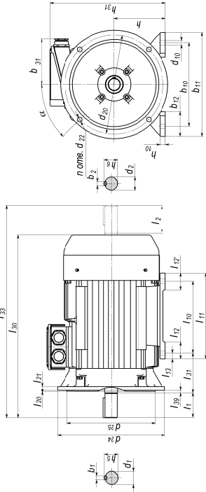
Привязка мощностей к установочно - присоединительным размерам по стандартам ГОСТ 31606 Power binding to mounting and overall dimensions according to GOST 31606
