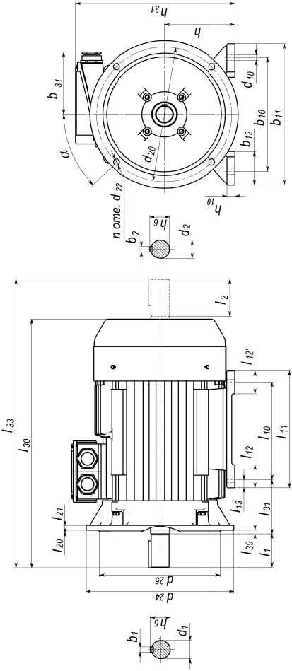
Габаритный чертёж IM 2001 (B35) / Dimension drawing IM 2001( B35)
