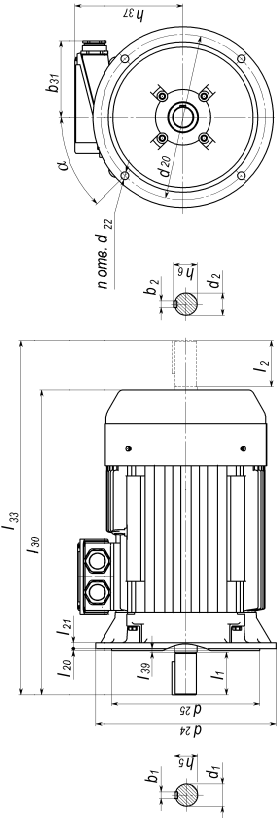
Привязка мощностей к установочно - присоединительным размерам по стандартам ГОСТ 31606 Power binding to mounting and overall dimensions according to GOST 31606
