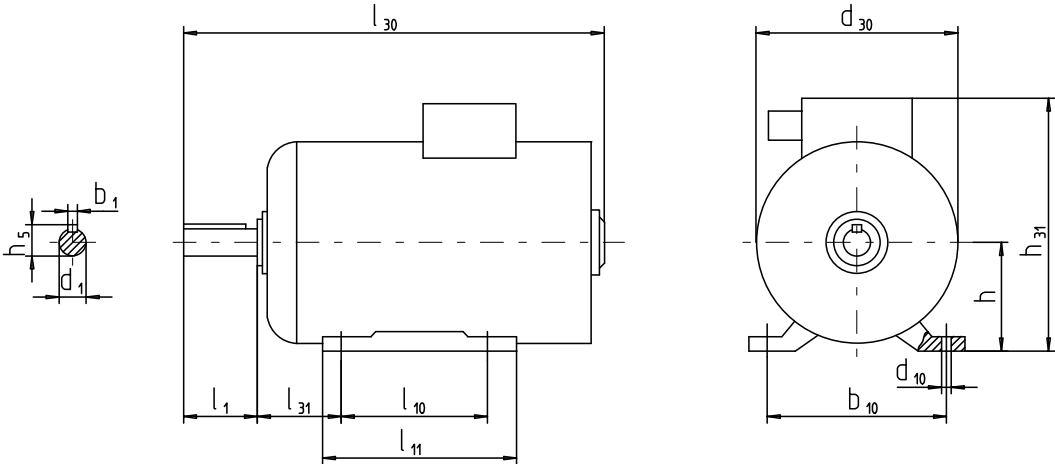
Размеры в мм. / Dimensions in mm.
