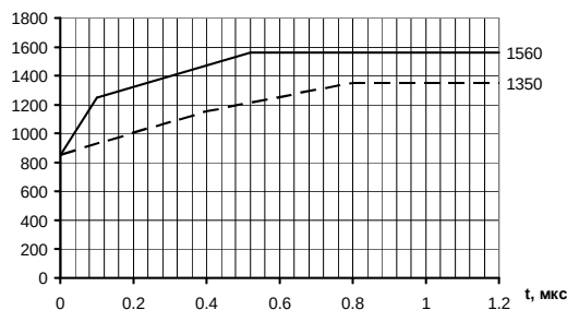
U_{max}, \text{В}
