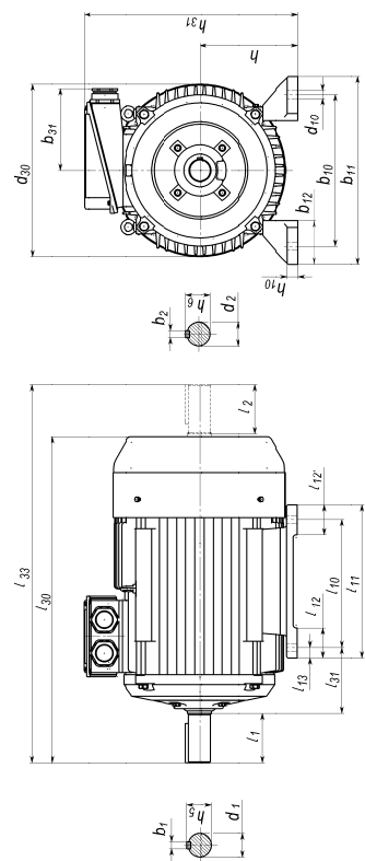
Привязка мощностей к установочно - присоединительным размерам по стандартам ГОСТ 31606 Power binding to mounting and overall dimensions according to GOST 31606 Размеры в мм / Dimensions in mm
