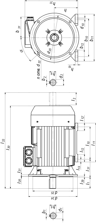
Привязка мощностей к установочно - присоединительным размерам по стандартам DIN EN 50347 Power binding to mounting and overall dimensions according to DIN EN 50347
