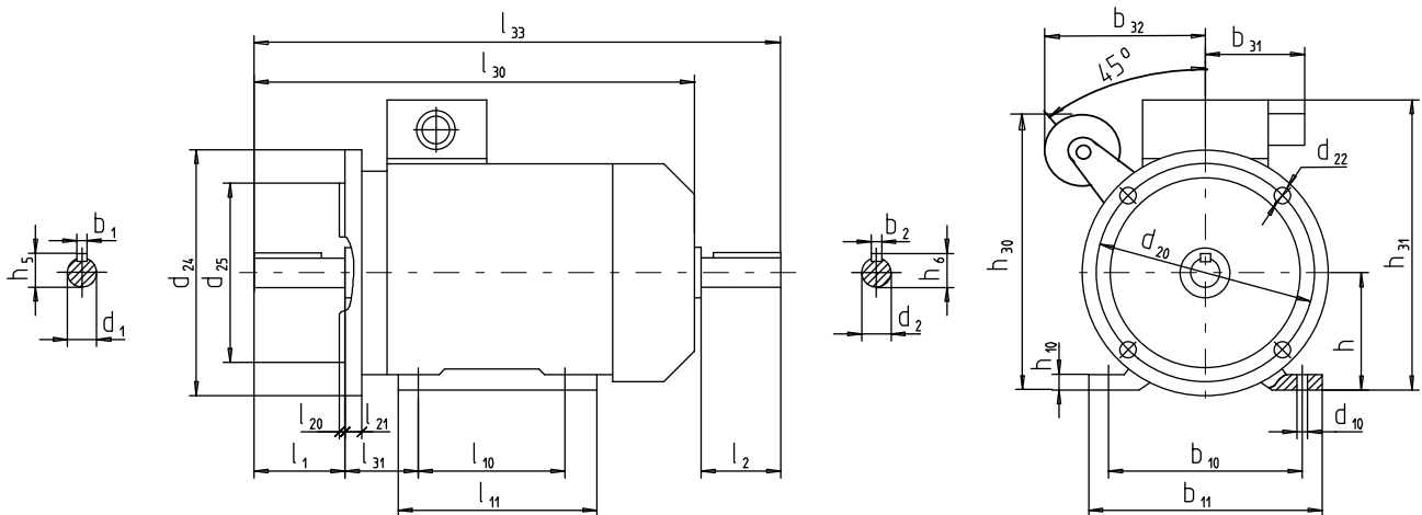
Размеры в мм /Dimensions in mm
